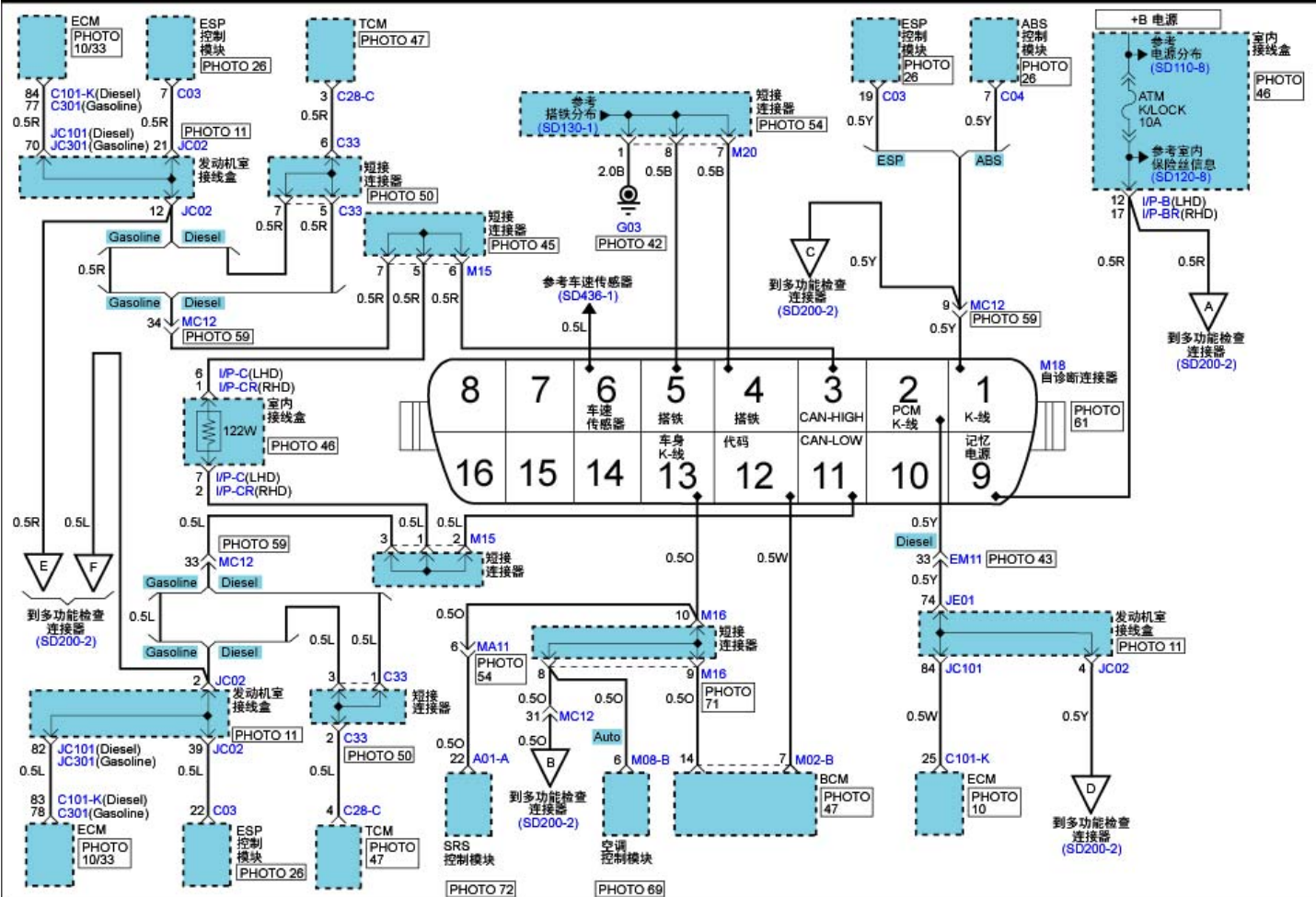
自诊断连接器(1)
